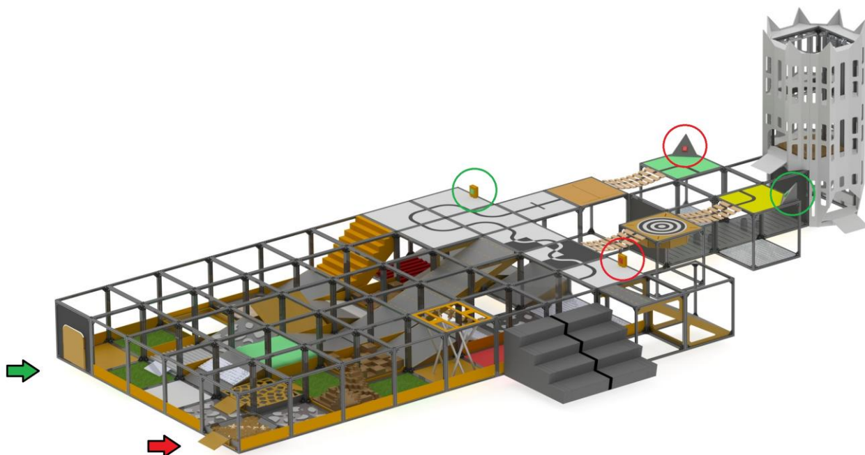
Рисунок 48 «Захват флага»
