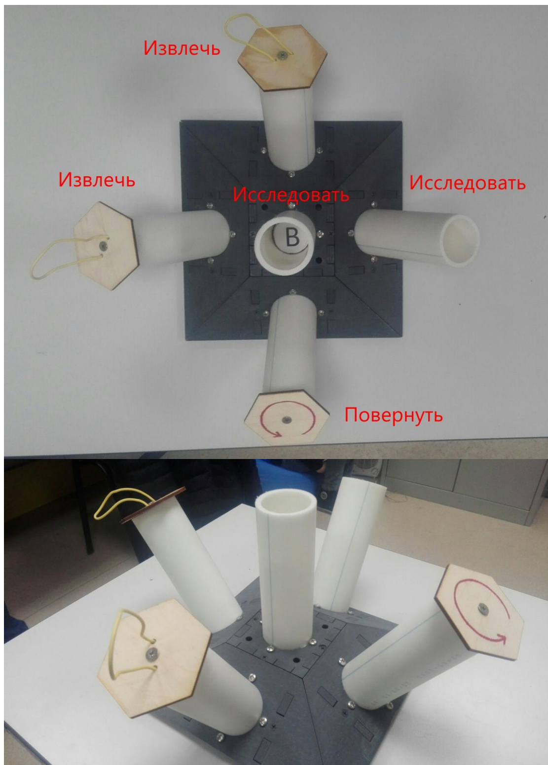
Рисунок 49 «Трубы»
