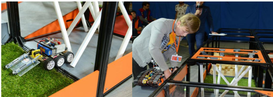
Рисунок 23 «Завал»
