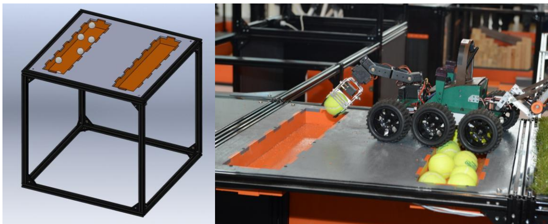
Рисунок 35 «Траншея»
