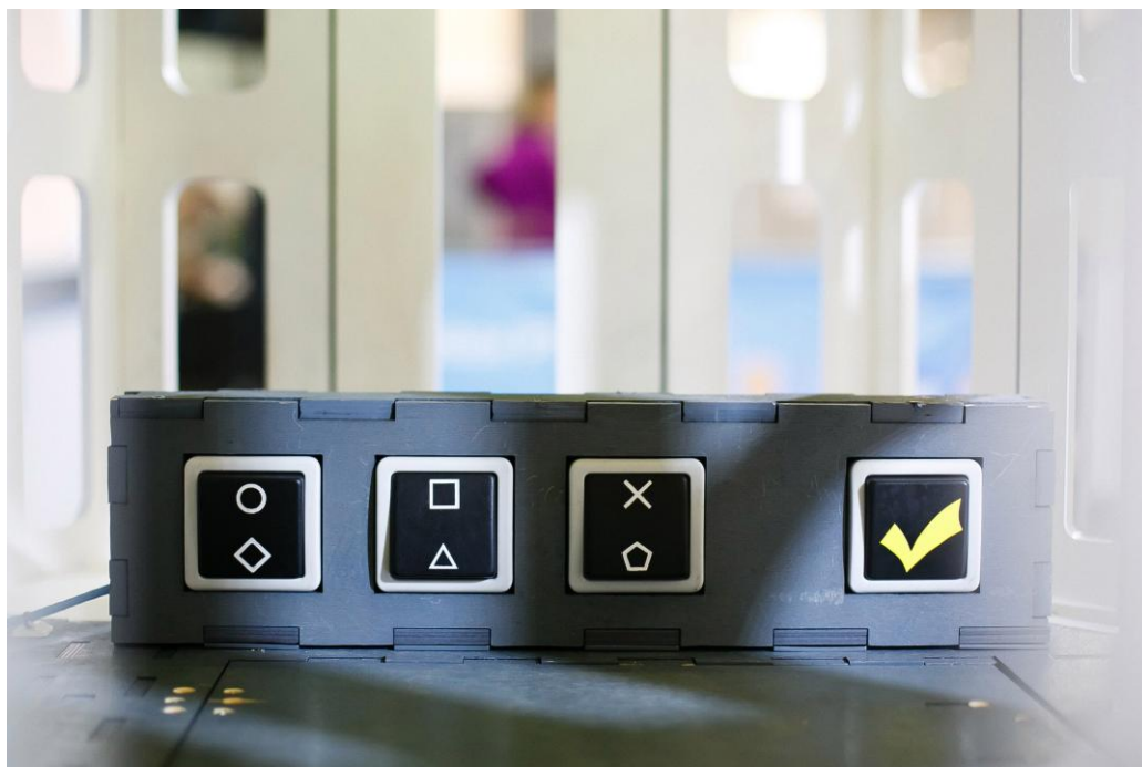
Рисунок 54 «Кнопки лифта»
