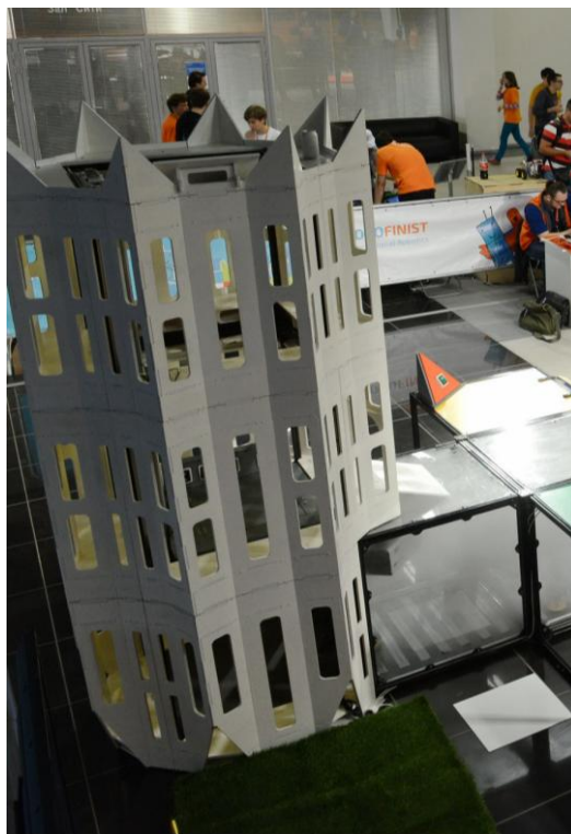
Рисунок 52 «Башня»
