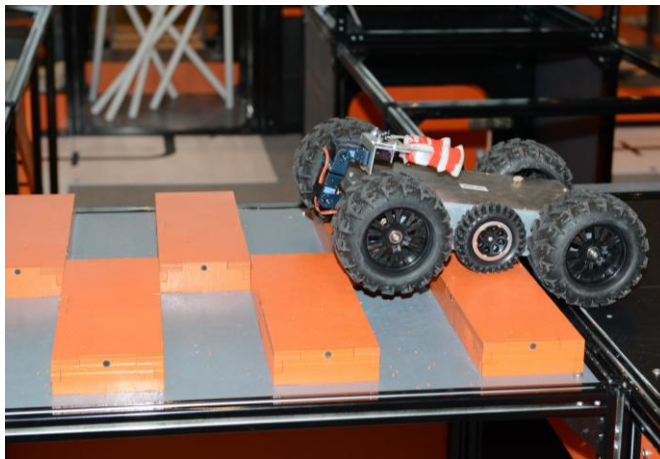
Рисунок 36 «Ребра»
