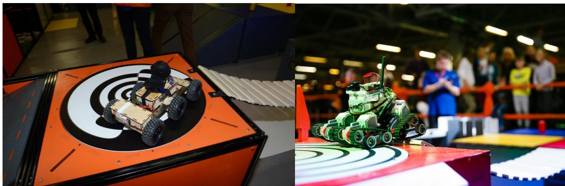
Рисунок 34 «Гипнодиск»
