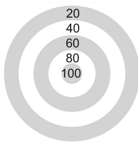
Рисунок 51 «Мишень»
