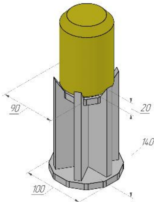
Рисунок 24 – «Башенка с маяком»
