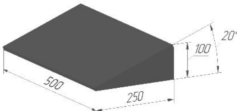
Рисунок 5 - «Наклонная поверхность лабиринта 20^\circ »
