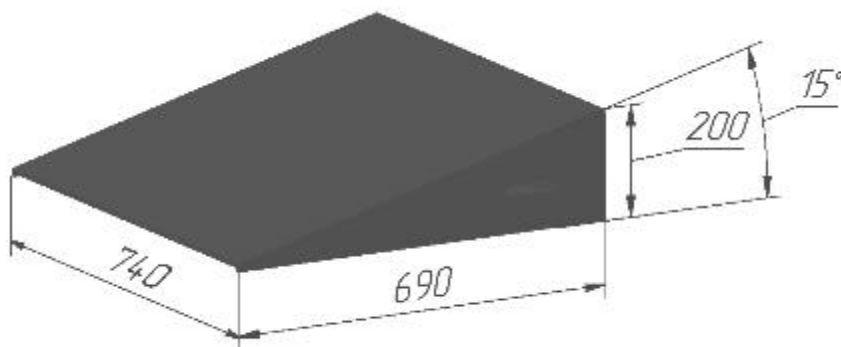
Рисунок 4 - «Наклонная поверхность лабиринта 15^\circ »
