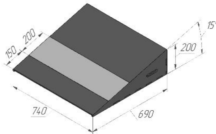
Рисунок 8 - «Скользкая наклонная поверхность лабиринта 15°»
