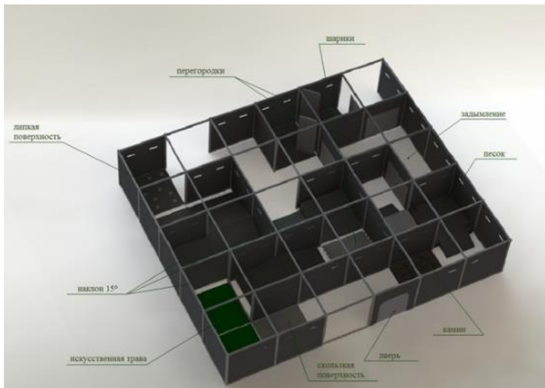
Рисунок 1 - «Пример сборки Лабиринта и размещения испытаний»
