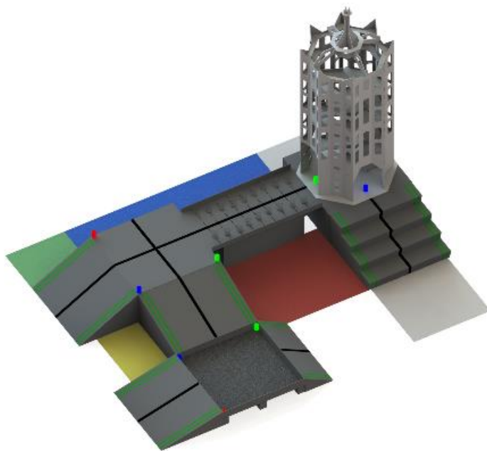
Рисунок 36 – «Пример расположения маяков на поле»
