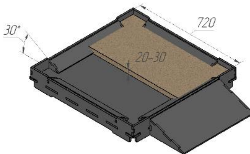
Рисунок 11 - «Короб с песком»
